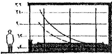
٣ - تزداد شدة الإضاءة مع ارتفاع فتحة الشباك (مقارنة ٢,١)
