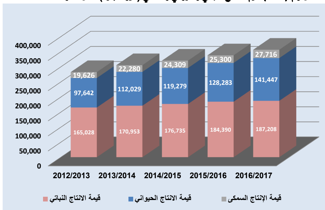
شكل رقم (2-24): قيم الانتاج النباتي والحيواني والسمكي (مليون جنيه) خلال الفترة 2012-2017
