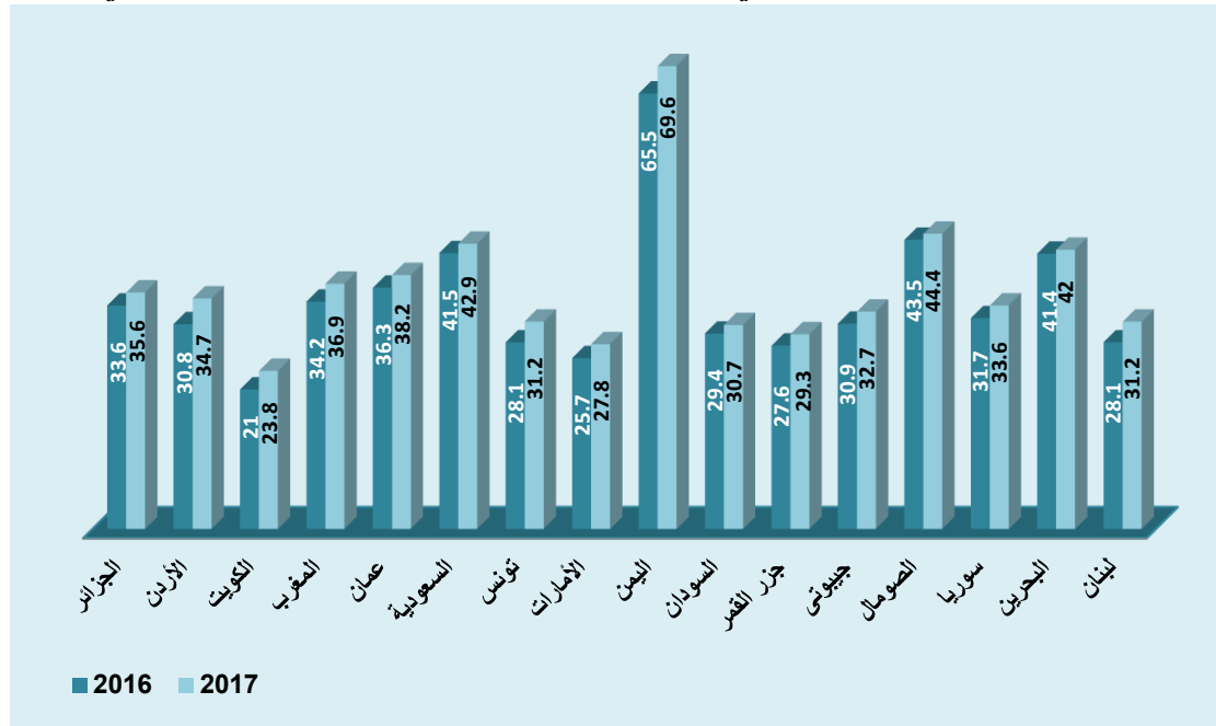
شكل رقم (1-19): نسب النساء في سن الإنجاب ويعانون من فقر الدم على المستوى العربي
