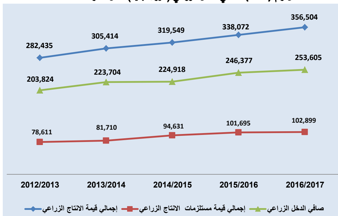
شكل رقم (2-25): صافي الدخل الزراعي (مليون جنيه) خلال الفترة 2012-2017
