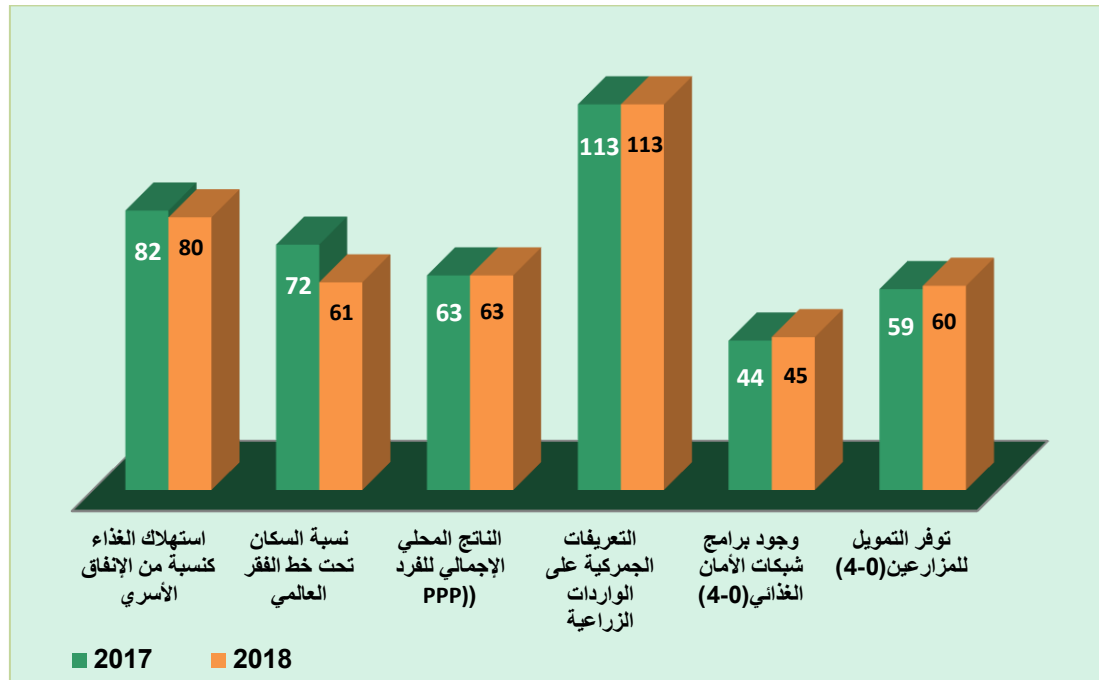
شكل رقم (2-3): ترتيب مصر على المؤشرات الفرعية
