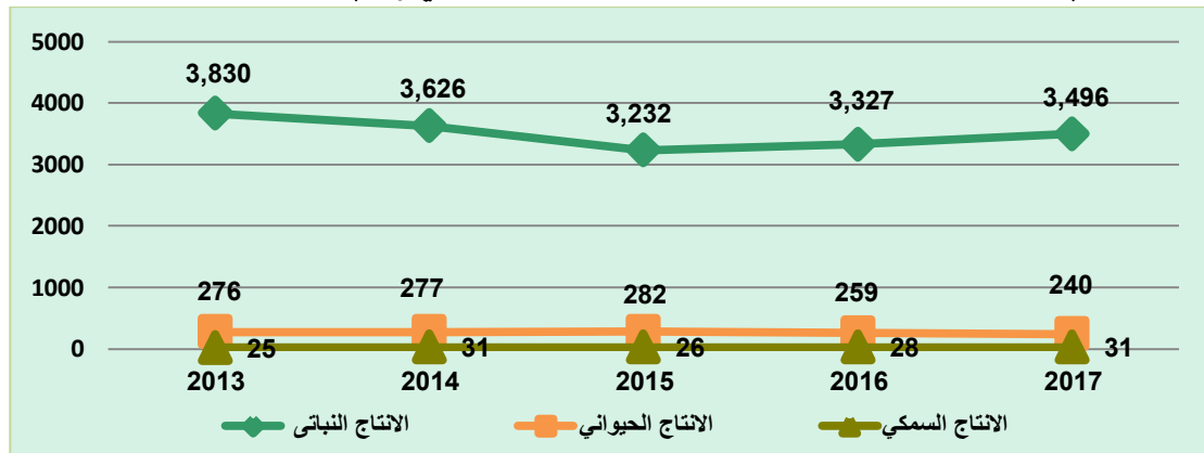
شكل رقم (3-22): متوسط نصيب الفرد السنوي من السعرات الحرارية/ يوم خلال الفترة 2013-2017
