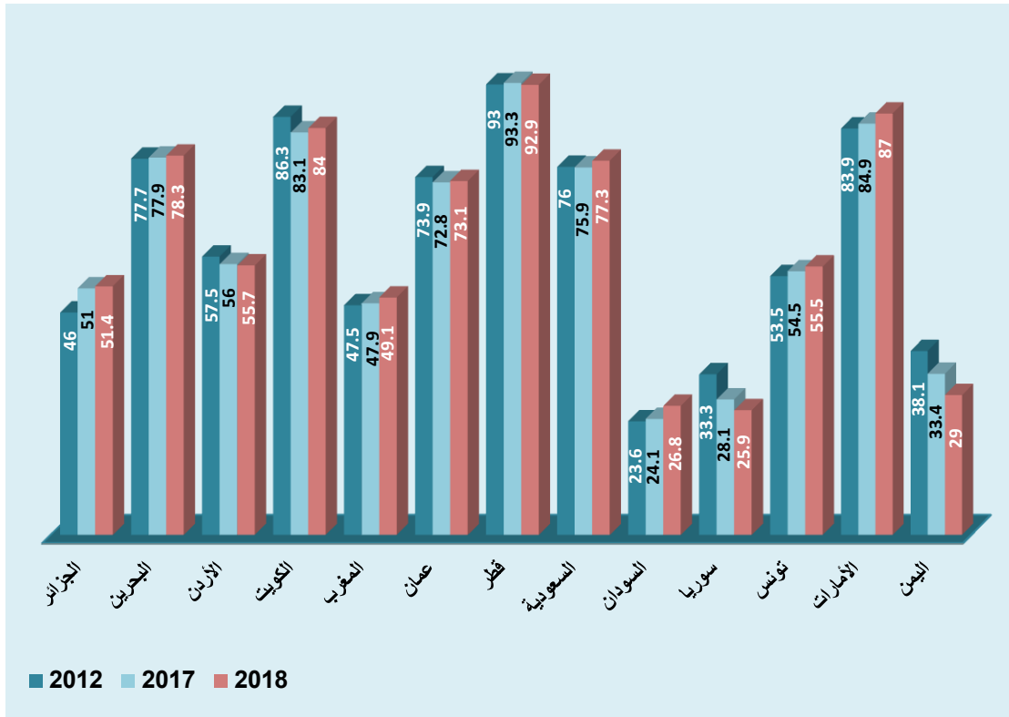
شكل رقم (1-8): مؤشر تحمل تكاليف الغذاء على مستوى الدول العربية خلال عام 2018 مقارنةً بعامي 2012، 2017
