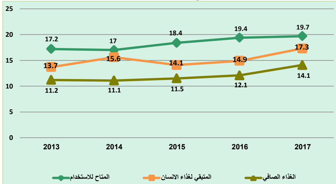
شكل رقم (3-8): كمية الغذاء الصافي من القمح (بالمليون طن) خلال الفترة 2017-2013
