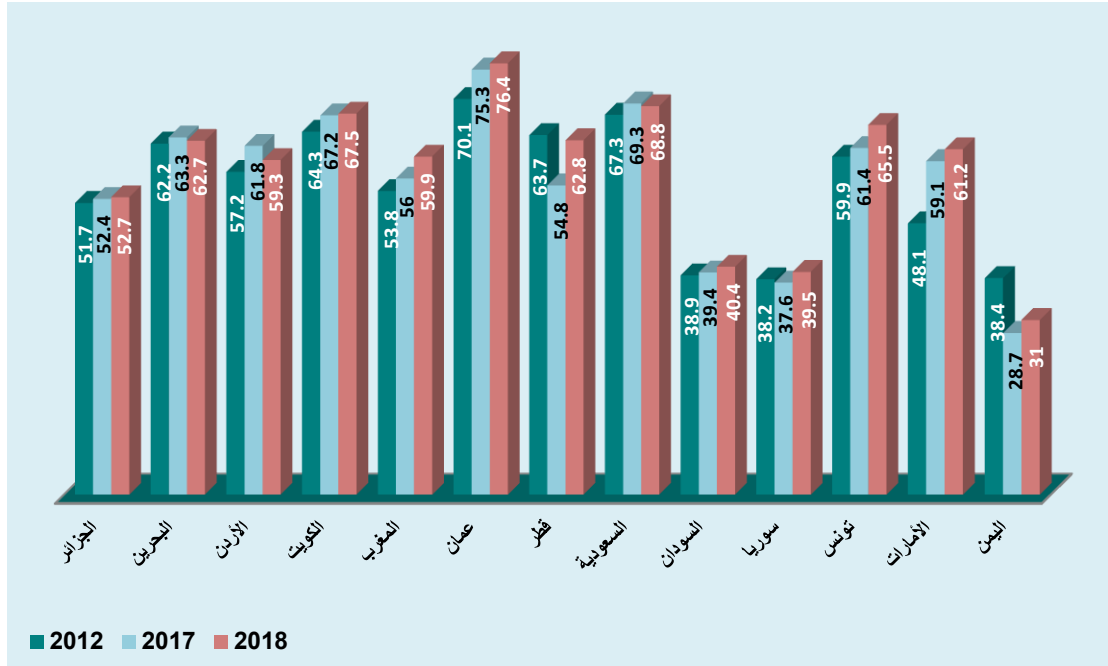
شكل رقم (1-9): مؤشر توافر الأغذية (الإتاحة) على مستوى الدول العربية خلال عام 2018 مقارنةً بعامي 2012، 2017
