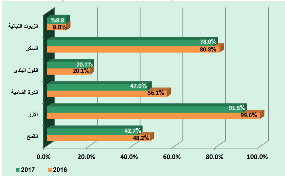
شكل رقم (3-6): نسب الإكتفاء الذاتي من أهم السلع النباتية خلال الفترة عامي 2016، 2017
