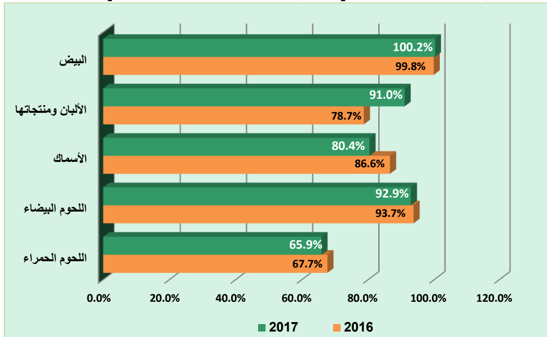
شكل رقم (3-7): نسب الإكتفاء الذاتي من أهم المنتجات الحيوانية خلال الفترة عامي 2016، 2017
