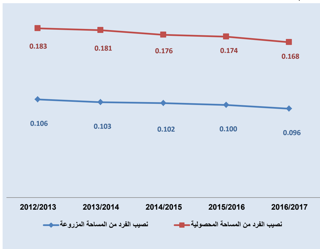
شكل رقم (6-2): نصيب الفرد من المساحات المنزرعة والمحصولية خلال الفترة 2017/2016-2013/2012
