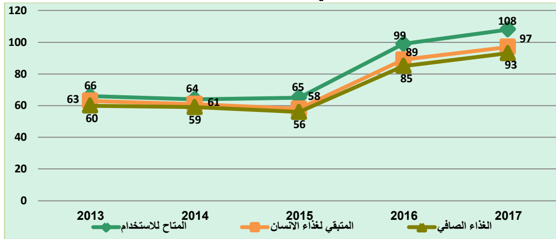
شكل رقم (3-11): كمية الغذاء الصافي من العنيس (بالألف طن) خلال الفترة 2013-2017
