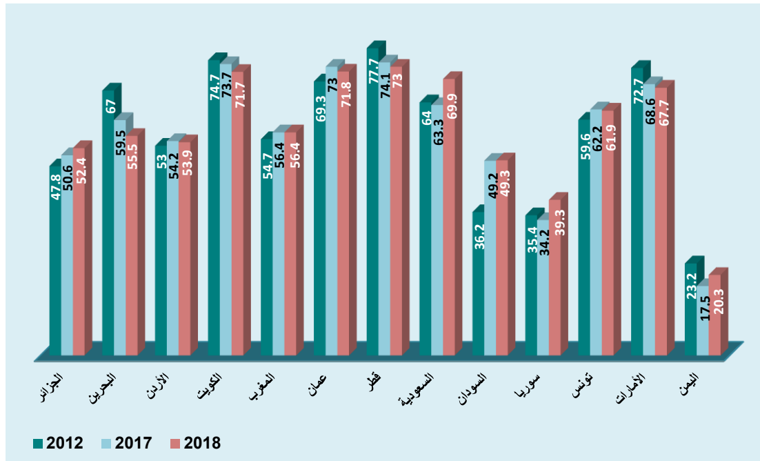
شكل رقم (1-10): مؤشر جودة وسلامة الغذاء على مستوى الدول العربية خلال عام 2018 مقارنةً بعامي 2012، 2017
