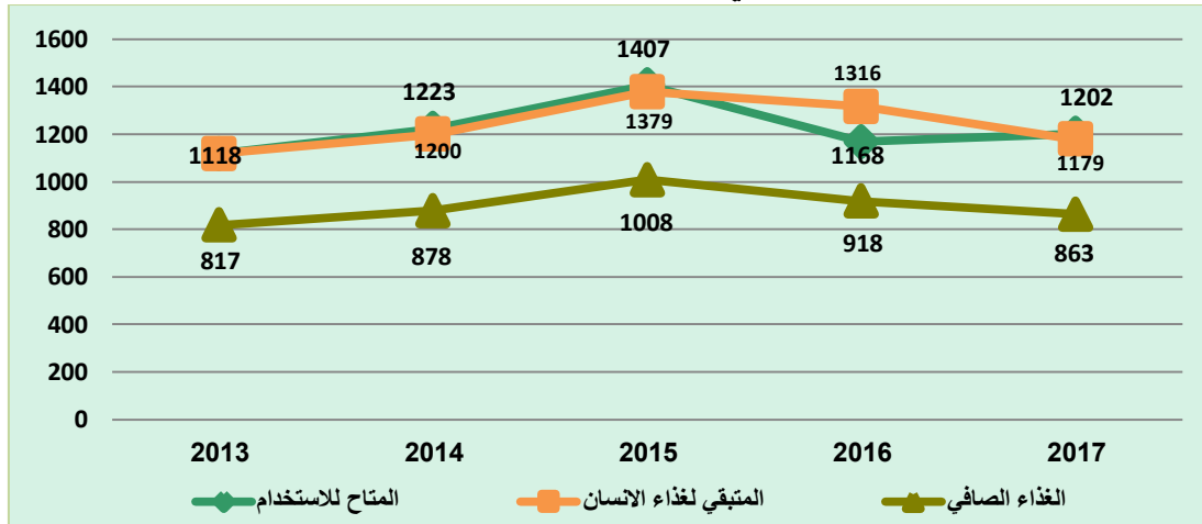
شكل رقم (3-15): كمية الغذاء الصافي من اللحوم الحمراء (بالآلف طن) خلال الفترة 2013-2017
