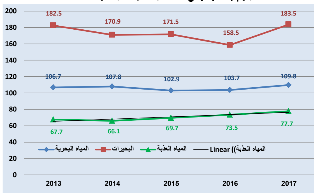
شكل رقم (2-22): إنتاج الأسماك بالمصايد خلال الفترة 2013-2017
