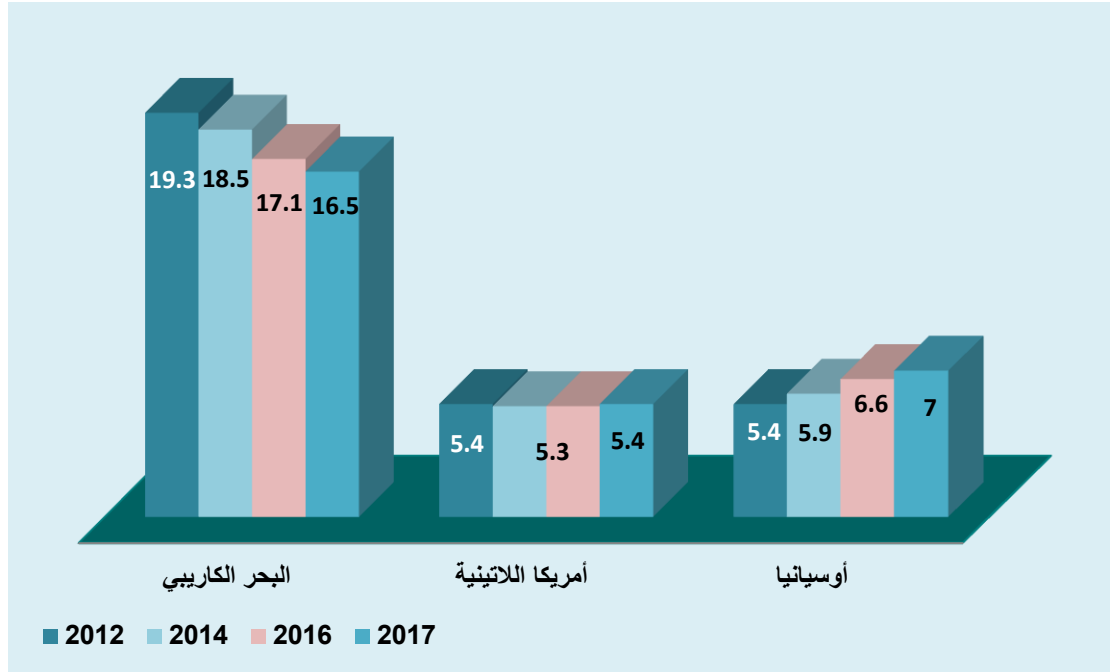
شكل رقم (1-15): نسب (%) انتشار نقص التغذية على مستوى أمريكا اللاتينية والبحر الكاريبي خلال الفترة 2012-2017
