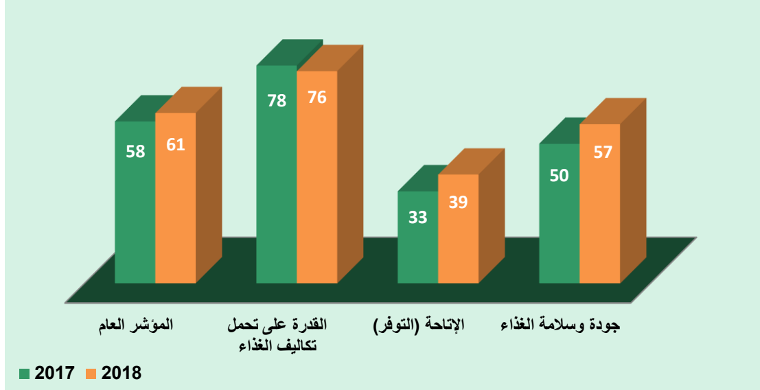
شكل رقم (3-1): ترتيب مصر على مؤشر الأمن الغذائي العالمي خلال عامي 2017-2018
