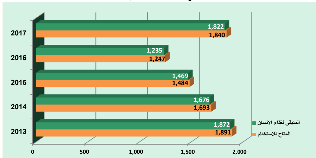
شكل رقم (3-12): كمية الغذاء الصافي من سكر القصب (بالألف طن) خلال الفترة 2013-2017
