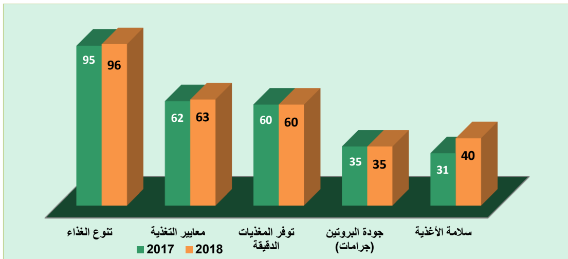
شكل رقم (4-3): ترتيب مصر على المؤشرات الفرعية لمؤشر جودة وسلامة الغذاء خلال عامي 2017-2018
