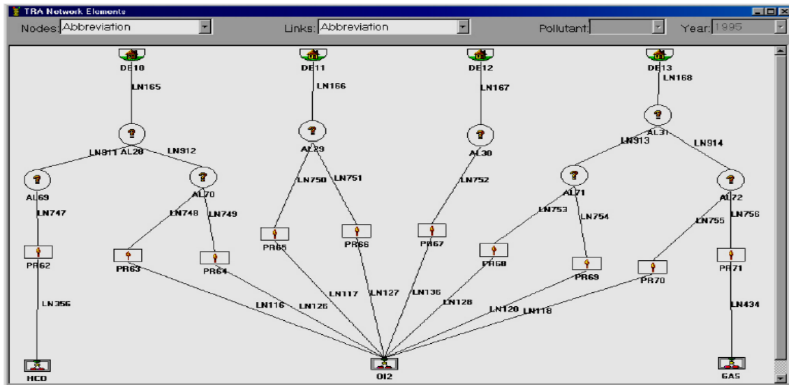
شكل (4-12): مثال لشبكة طاقة بسيطة
