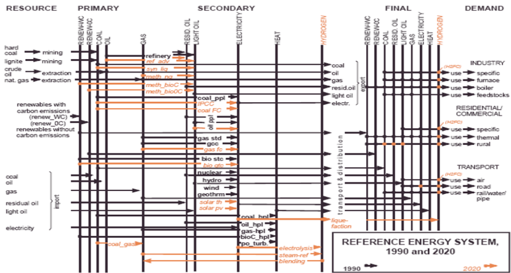
شكل (3-4): مرجعية نظام الطاقة لنموذج MESSAGE
