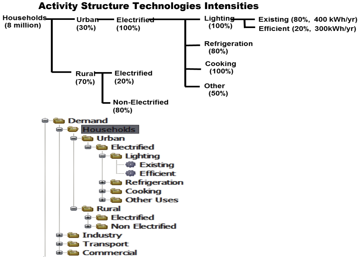
شكل (4-9): مثال لشجرة توضح نمذجة الطلب علي الطاقة
