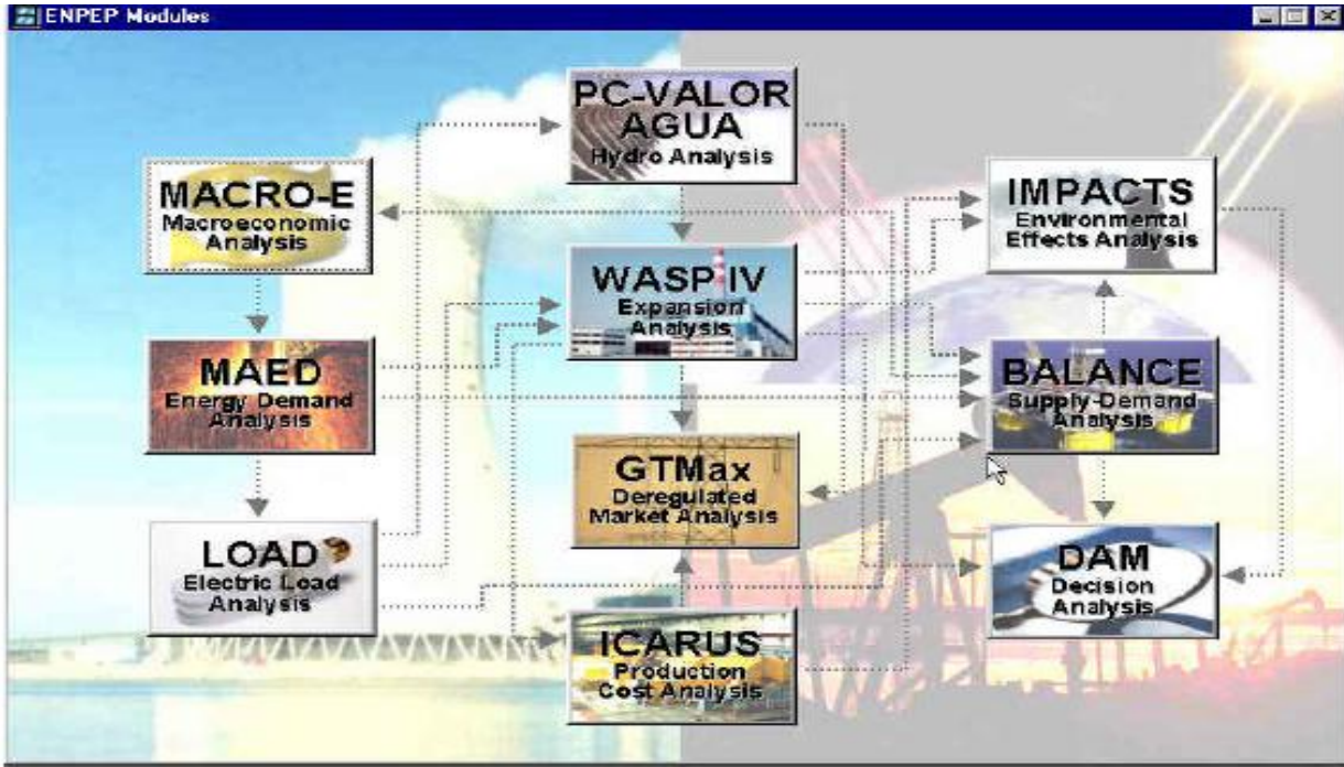
شكل (4-10): مكونات نموذج ENPEP
