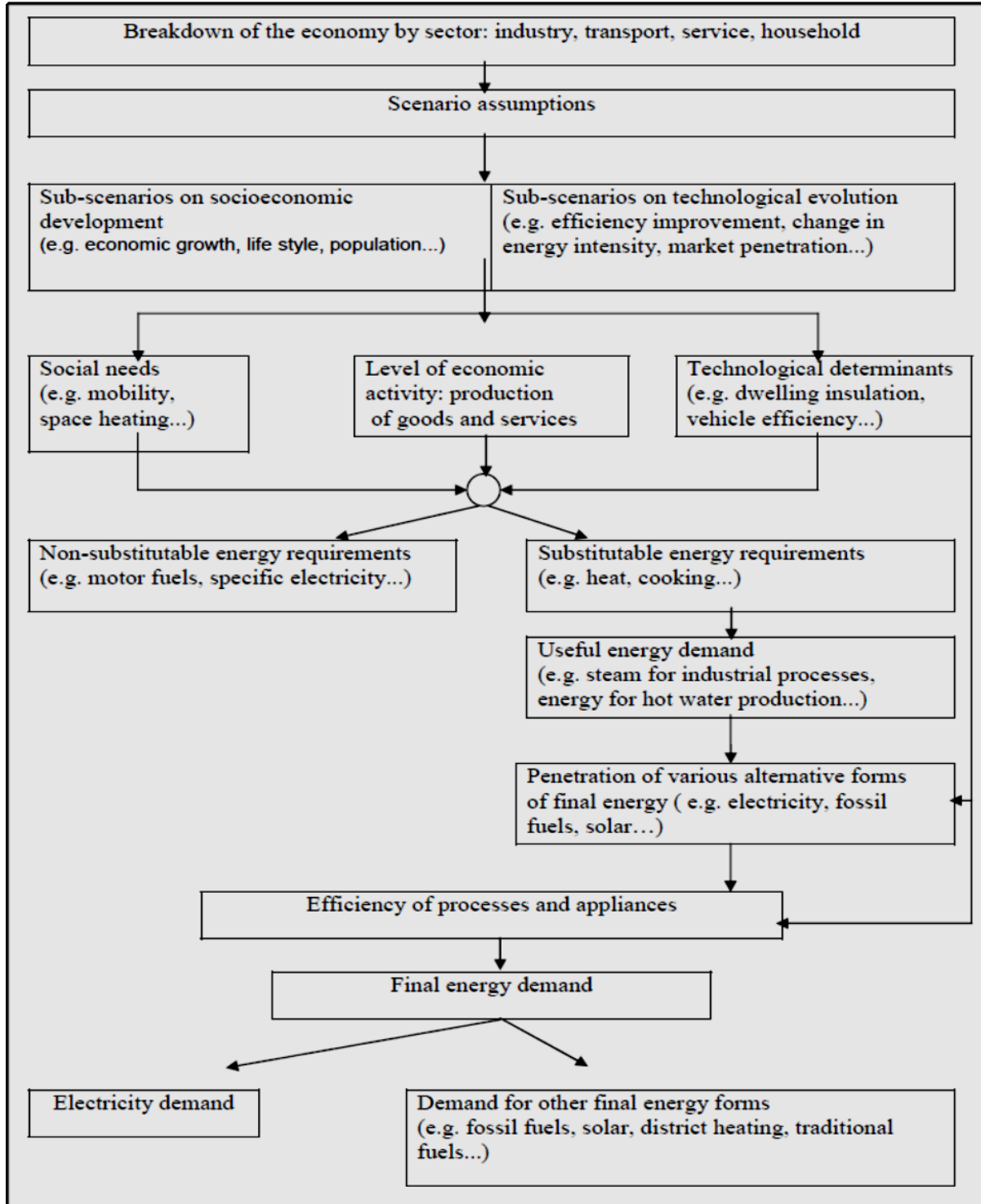
شكل (4-1): الإطار العام للتحليل المستخدم في إسقاط الطلب علي الطاقة باستخدام نموذج MAED
